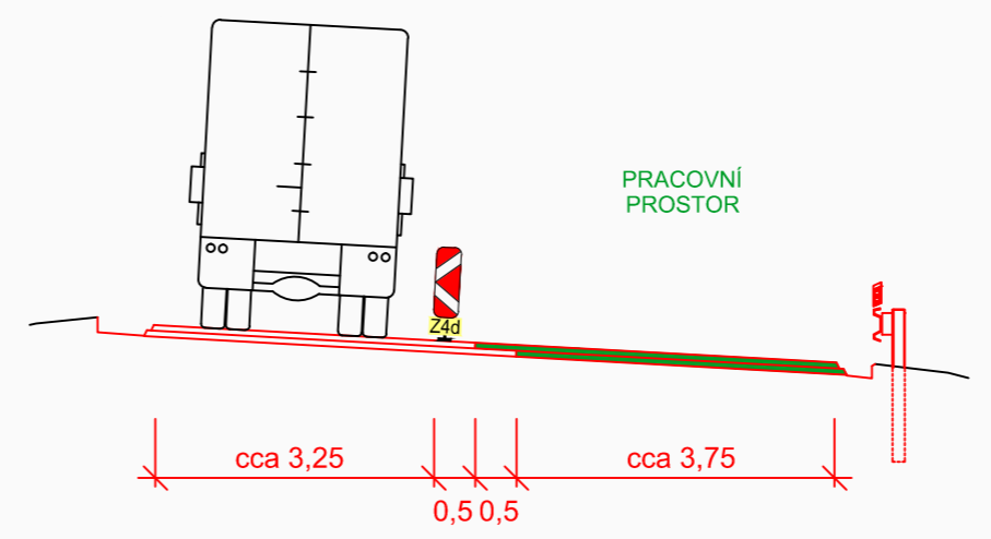
ŠÍŘKOVÉ USPOŘADÁNÍ NA VĚTVI 1:100
